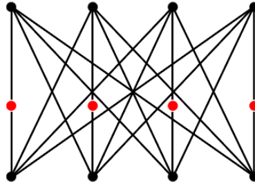
K_{4,4} +一组完美匹配进行 Subdivision
