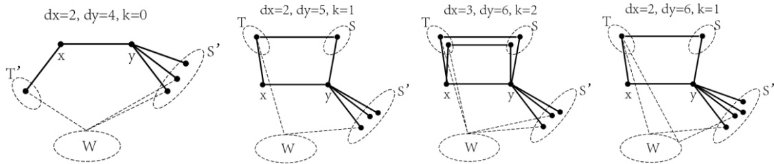
图 6: 引理 9, 两 endpoint 度数相差超过 2 或者度数差和度数-4 圈数都 \geq 2 , 边 Ricci 曲率=0
